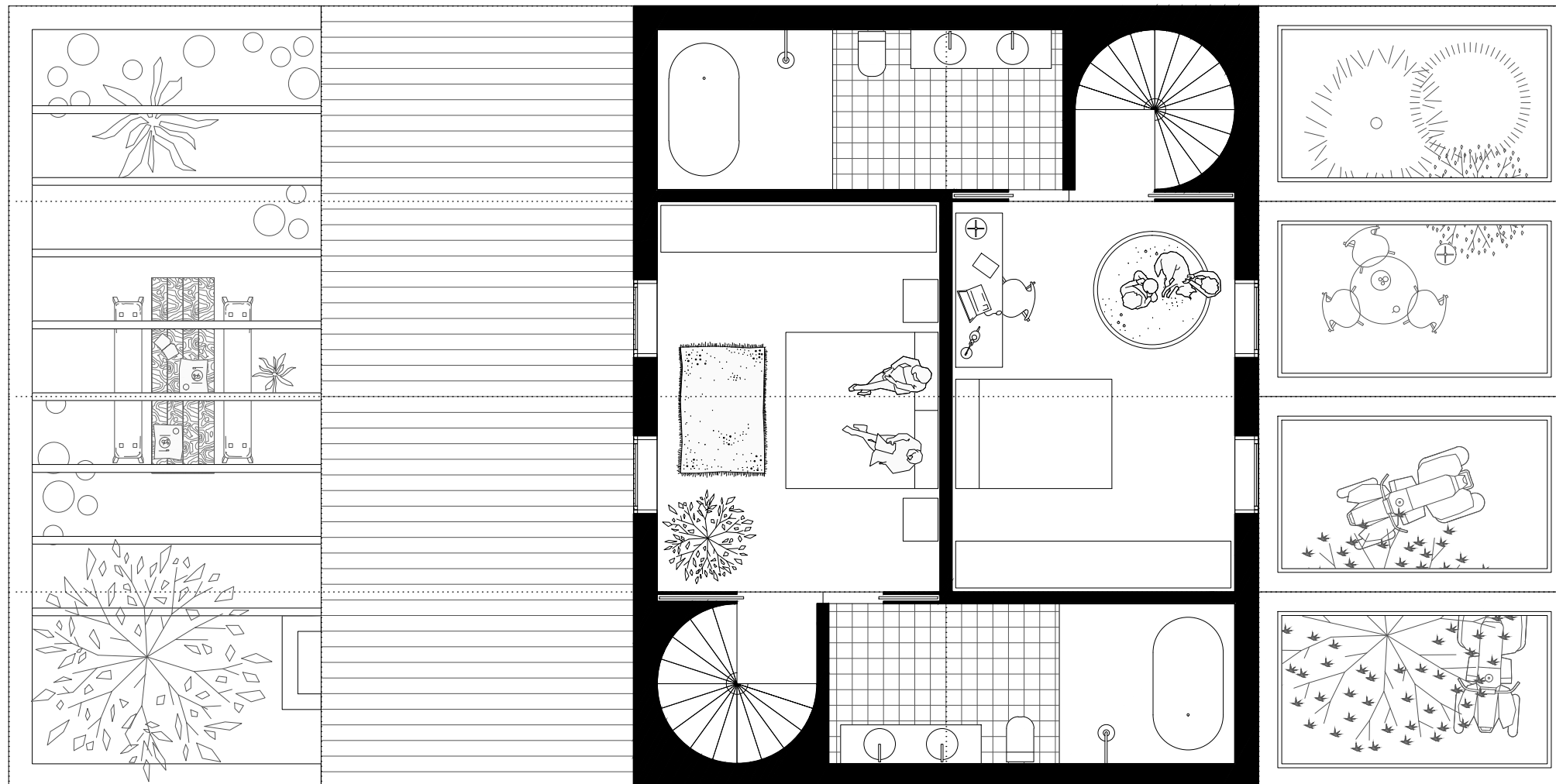
🕒 PLANTA SEGONA E 1.75
