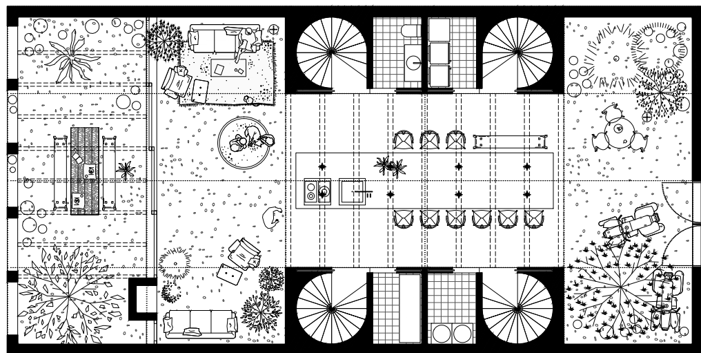
🕒 PLANTES I SECCIONS PROPOSTA CASA UNIFAMILIAR AMB 4 HABITACIONS E 1.150
